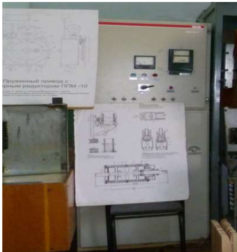
Рис.9. Зовнішній вигляд лабораторного стенду №5 з демонстративними матеріалами для вивчення конструкції дугогасної камери елегазових, вакуумних високовольтних вимикачів та демонстрації роботи комплектної комірки 10 кВ з вакуумним вимикачем серії ВР-10 кВ
